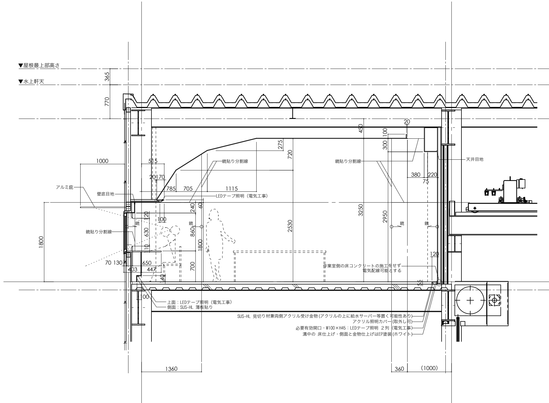
矩計図(1) S=1:50
